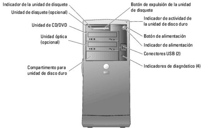
Figura 1-1. Características e indicadores del panel frontal
